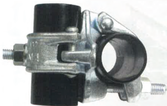
▲ DF 403 DOUBLE COUPLER (EN-74 / BS-1139)
